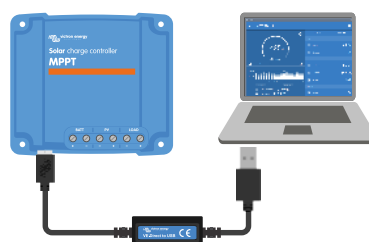
Connexion à l'application VictronConnect à travers l'USB en utilisant une interface VE.Direct-USB
